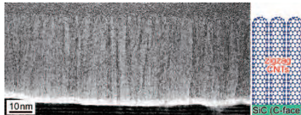
CNTの電子顕微鏡写真 先端にキャップをもち、直径約3nm、長さ約30nmのCNTが高密度に配向して形成されている。
