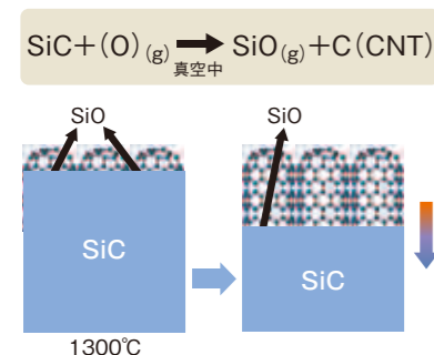
SiC結晶を真空中、高温で熱処理することにより、Si原子が除去され、残存したC原子がCNTを形成。
