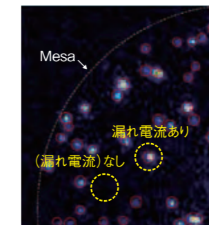
エミッション像 電流の漏れが発光点となって観察される一部の欠陥のみが発光点と重なる
