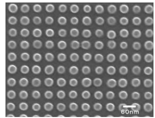
電子線描画によるナノパターン形成 Nano-pattern by EB lithography
