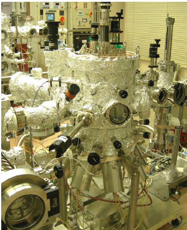
8元マグネトロンスパッタ装置 Magnetron sputtering with 8 sources
