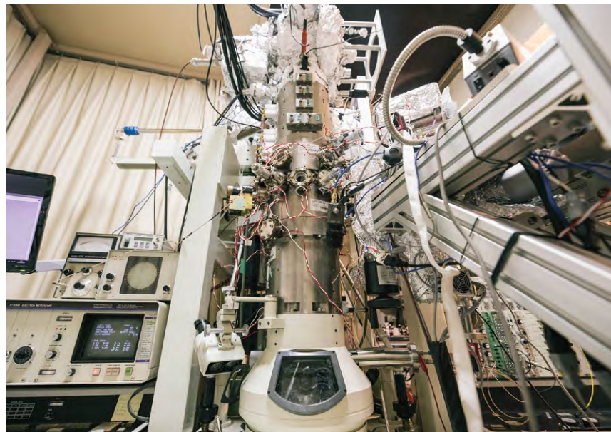
本研究グループで開発したスピン偏極パルス電子顕微鏡 Spin-polarized ultrafast transmission electron microscope developed by our group
