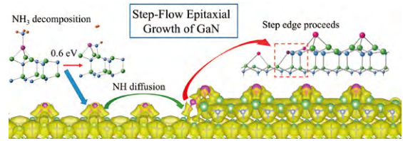
量子論第一原理計算によるGaNエピタキシャル成長素過程の解明 表面ステップ端の黄色い電子雲の切れ目からNが膜中に取り込まれる
