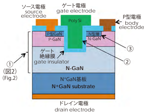
図1. 縦型トレンチGaNデバイス Fig.1 A Vertical trench GaN device
