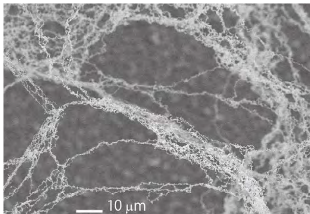
ヘリウムプラズマ照射により形成されたタングステンナノワイヤー Tungsten nanowires grown by an exposure to a helium plasma.
