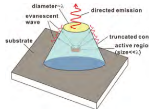
エバネッセント光の結合効果を利用した指向性LEDの模式図
