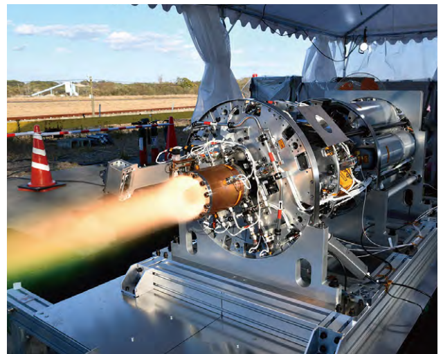
デトネーション推進システムの宇宙フライトモデル Space flight model of detonation propulsion system
