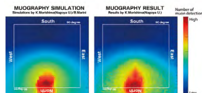
素粒子ミューオンを使った計測のシミュレーションと測定結果の比較 Comparison of muography simulation and results for descending corridor
