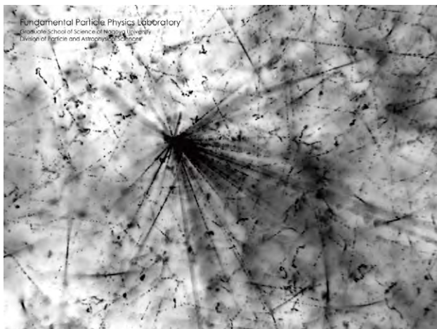
高エネルギーの宇宙線が乳剤中の原子と衝突して起こった反応をとらえた顕微鏡写真 This micrograph showing the reaction that occurred when high-energy cosmic rays collided with atoms in the emulsion.
